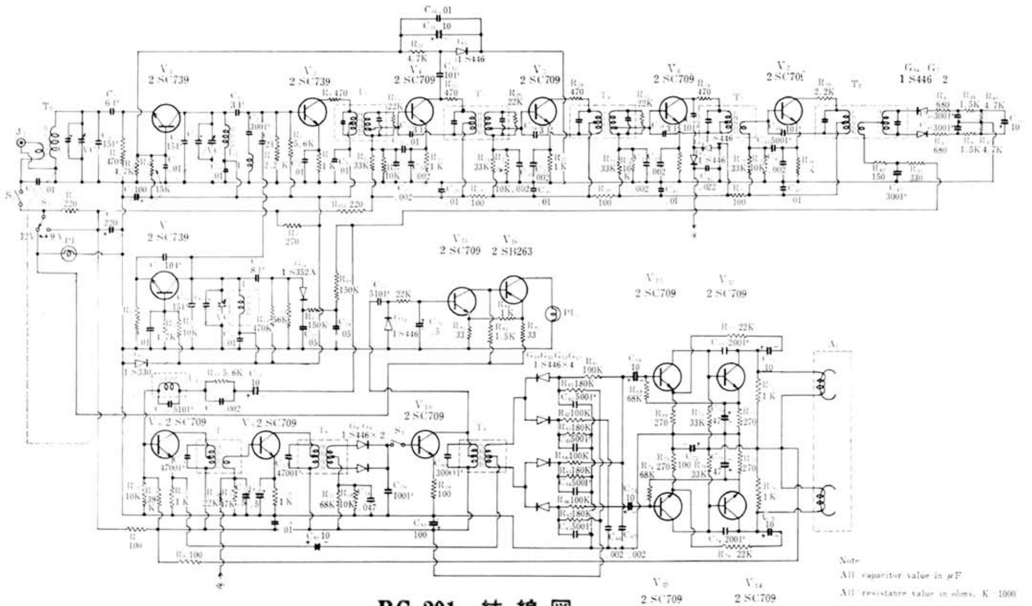
RC-201 結線図
