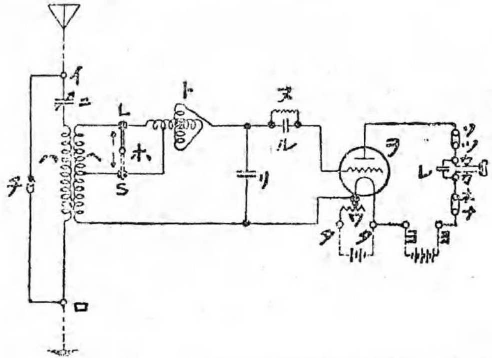
一トムフォン「二號型受信機 接續圖
