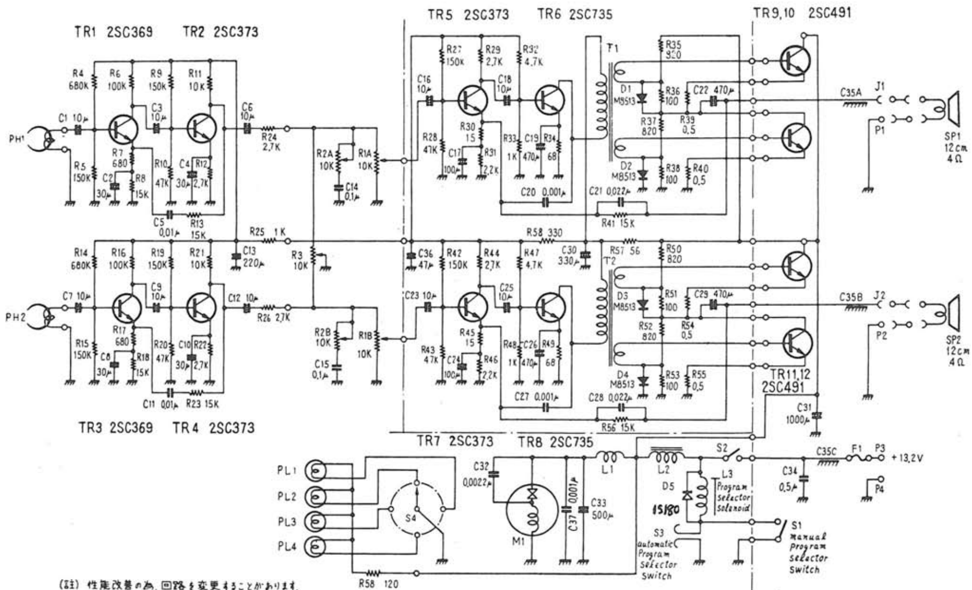
「東芝」KT-82C回路図
