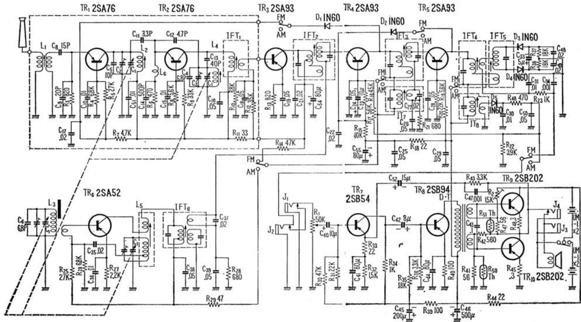
東芝 10 TL-429 FAY 形 10石 FM/AM トランジスタラジオの回路
