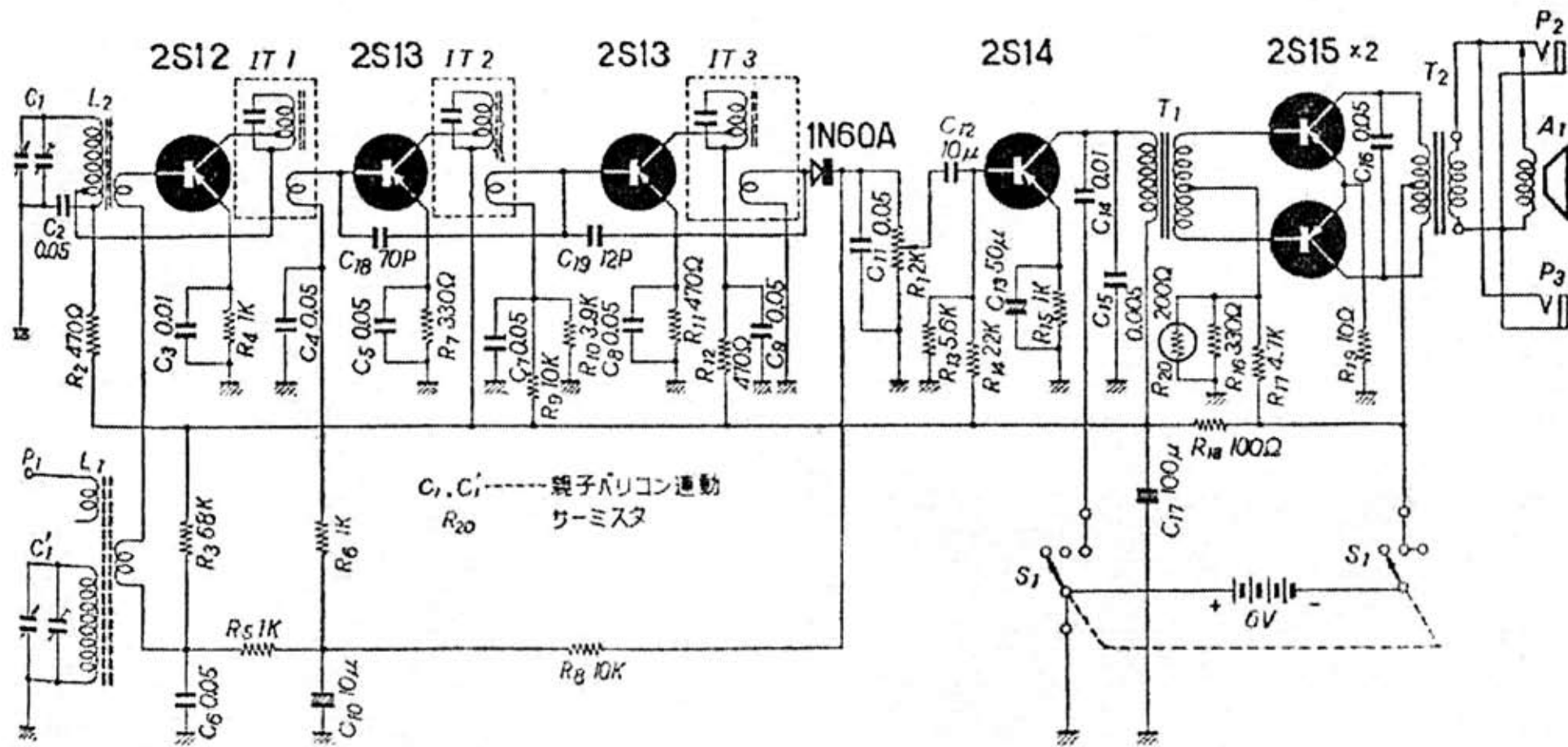
6 TR-127 型 6 石ラジオの全回路図
