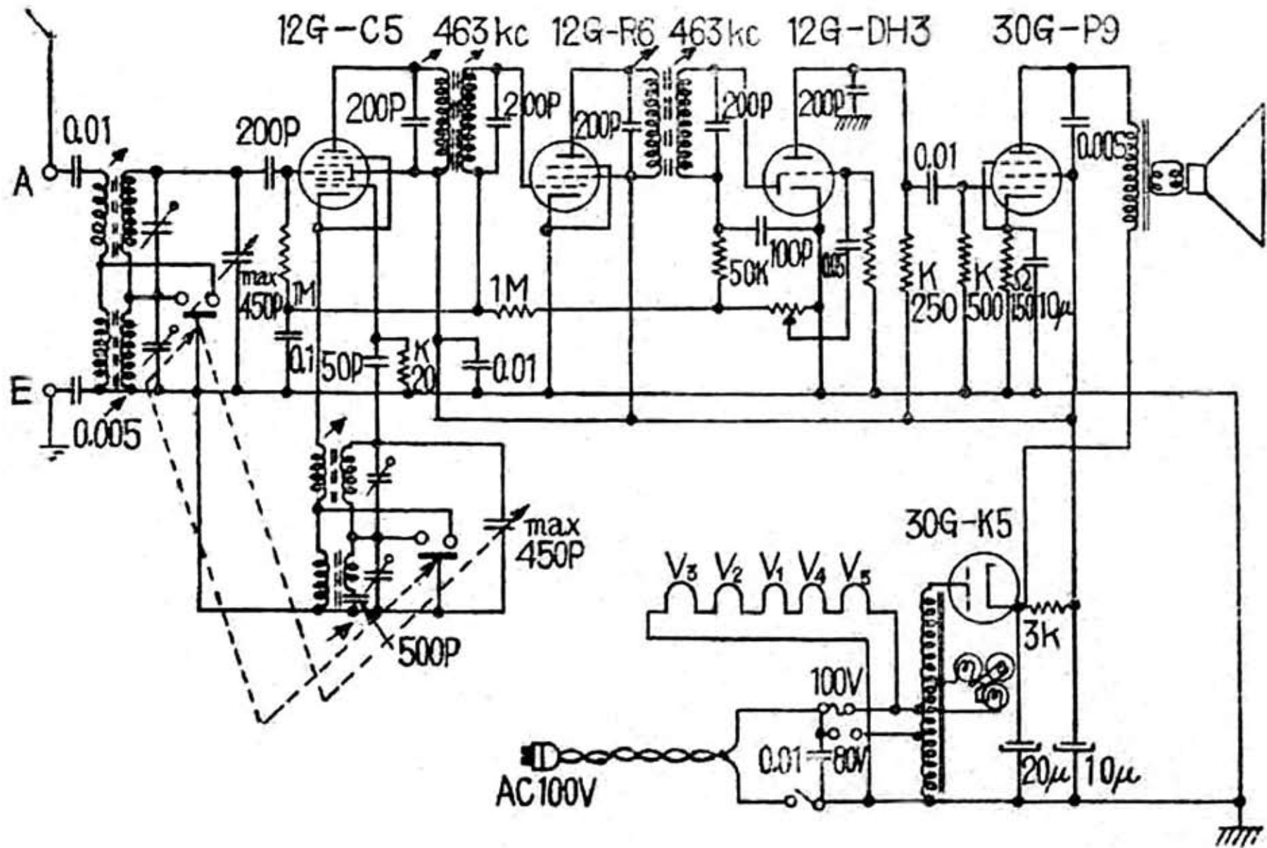
五球全波受信機の接続図
