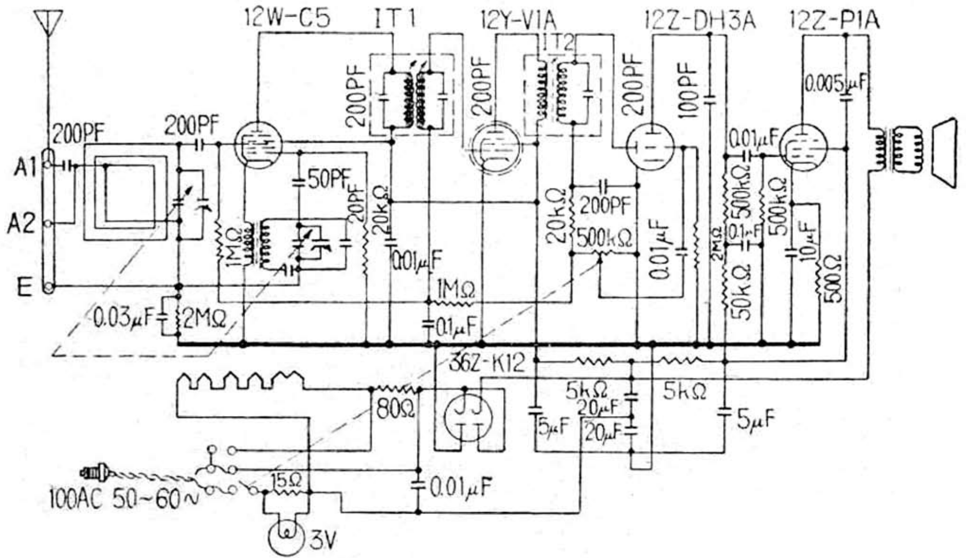
ZS-1056 受信回路
