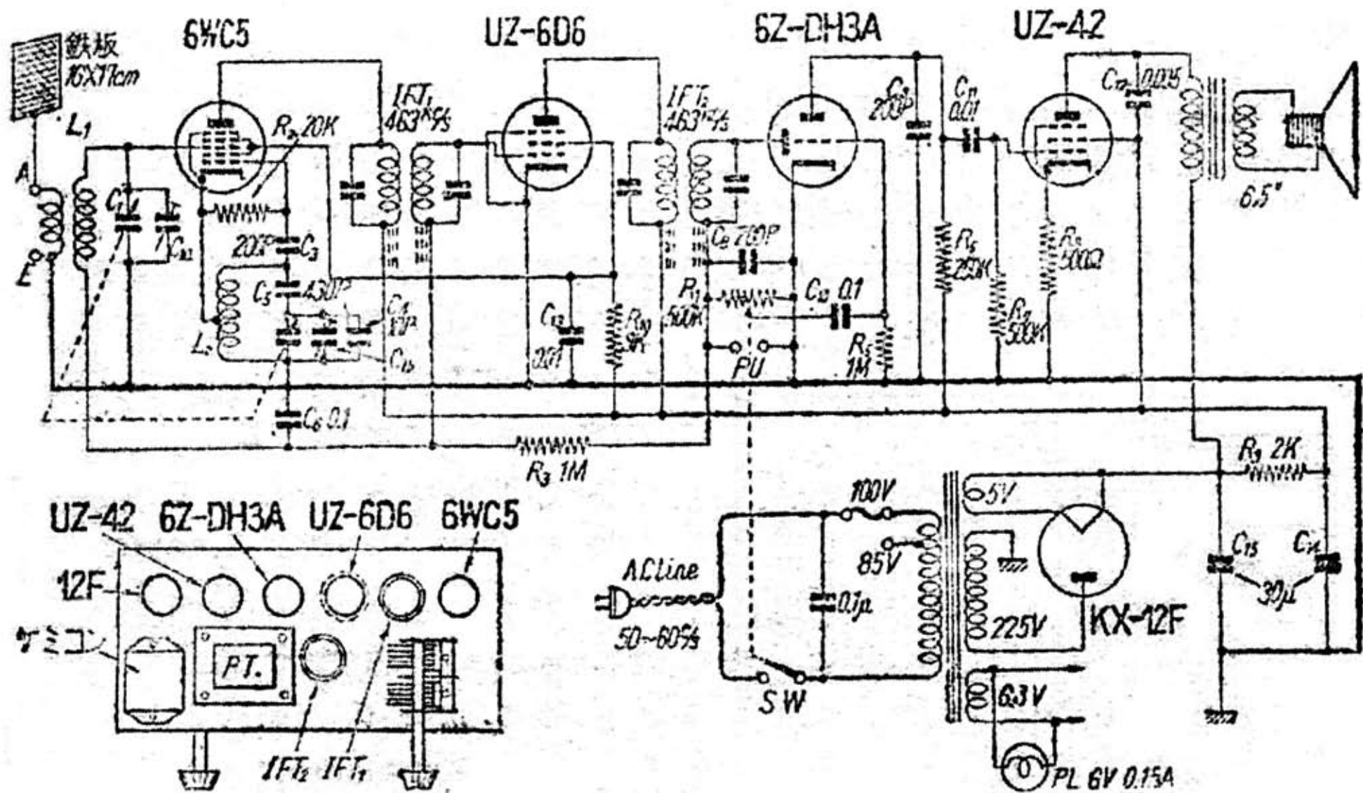
東京芝浦電気製“マツダ ZS-1130”型5球スーパー回路図および部品配置図
