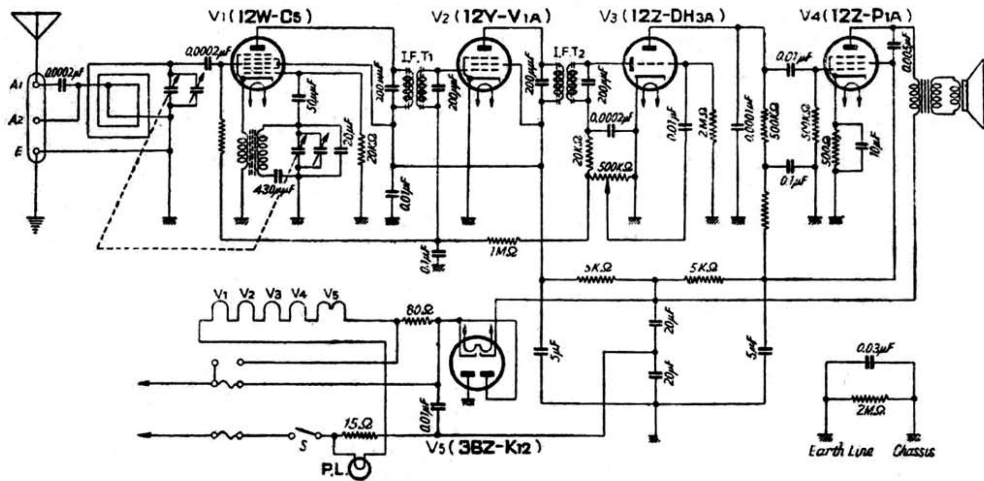
東京芝浦電気製[ホームスーパー]5球式スーパーヘテロダイン受信機
