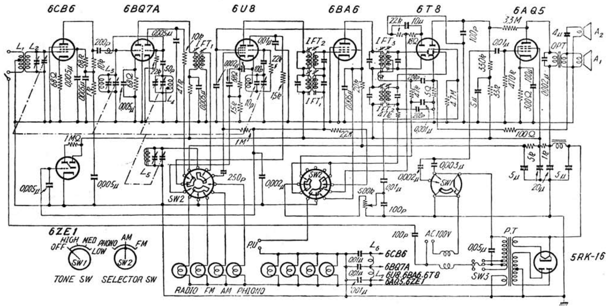
マ ツ ダ 7AF-100 型 受信機 の 回路 図
