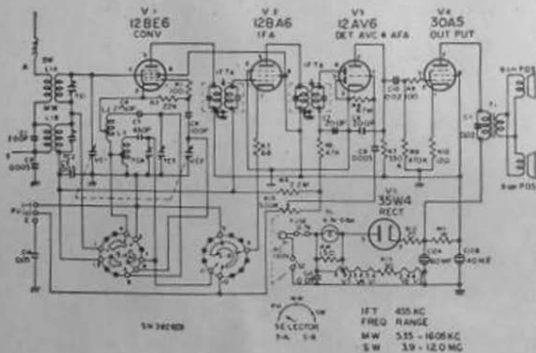
配線図
