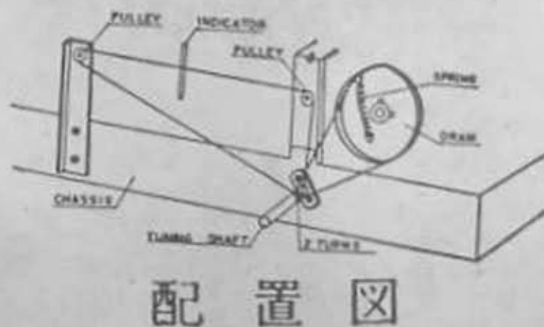
糸掛図
