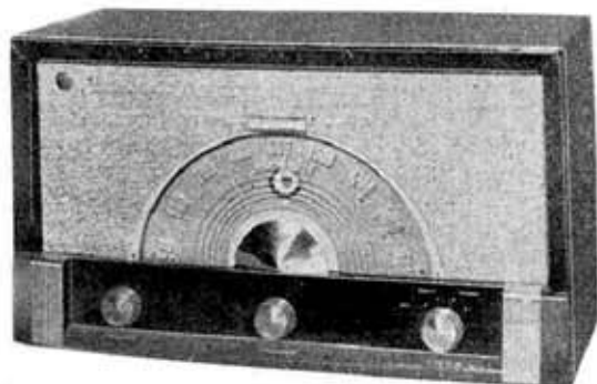
第 10.22 図 マツダラジオ 611 A 型 Matsuda radio receiver 6 tube super heterodyne, type 611 A
