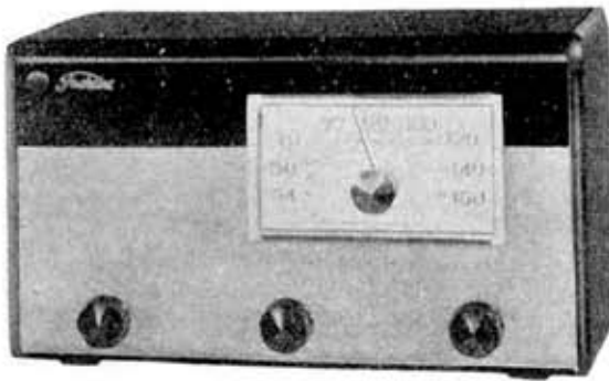
第 10.14 図 マツダラジオ 513 D 型 Matsuda radio receiver, 5 tube super heterodyne, type 513 D
