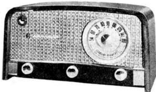
第 10.21 図 マツダラジオ 614 A 型 Matsuda radio receiver, 6 tube super heterodyne, type 614 A
