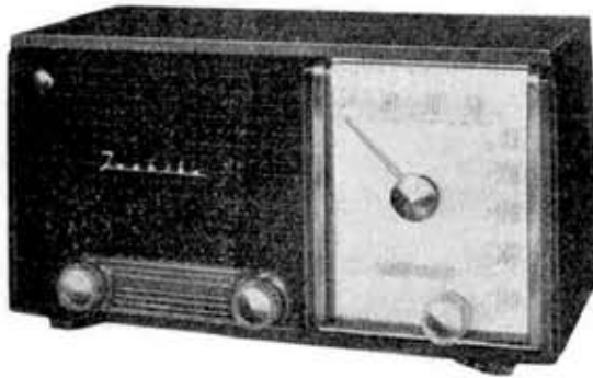
第 10.15 図 マツダラジオ 513 E 型 Matsuda radio receiver, 5 tube super heterodyne, type 513 E
