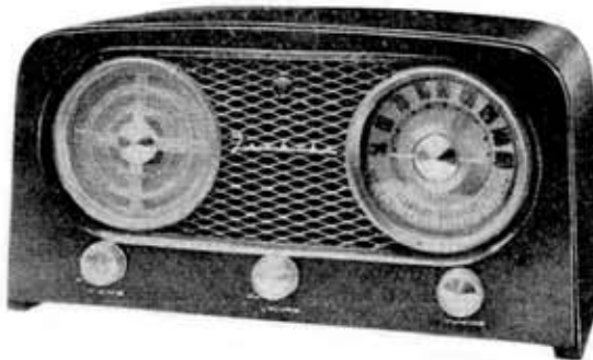
第 10.16 図 マツダラジオ 513 F 型 Matsuda radio receiver 5 tube super heterodyne, type 513 F
