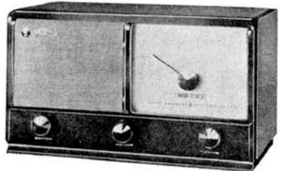
第 10.17 図 マツダラジオ 514 A 型 Matsuda radio receiver, 5 tube super heterodyne, type 514 A
