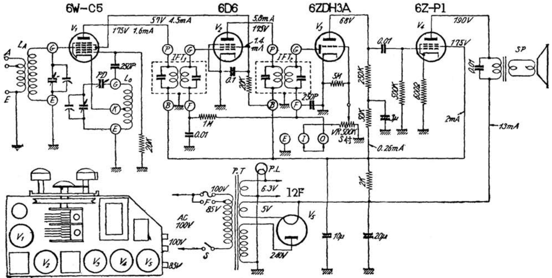
MS-5C 型スーパーヘテロダイナ配線図
