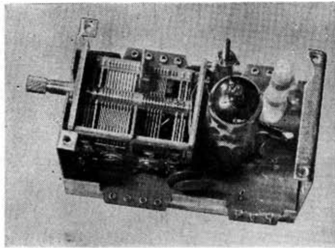
バリコン同調 FM フロントバック, トリオ AFP-UA-W 形
