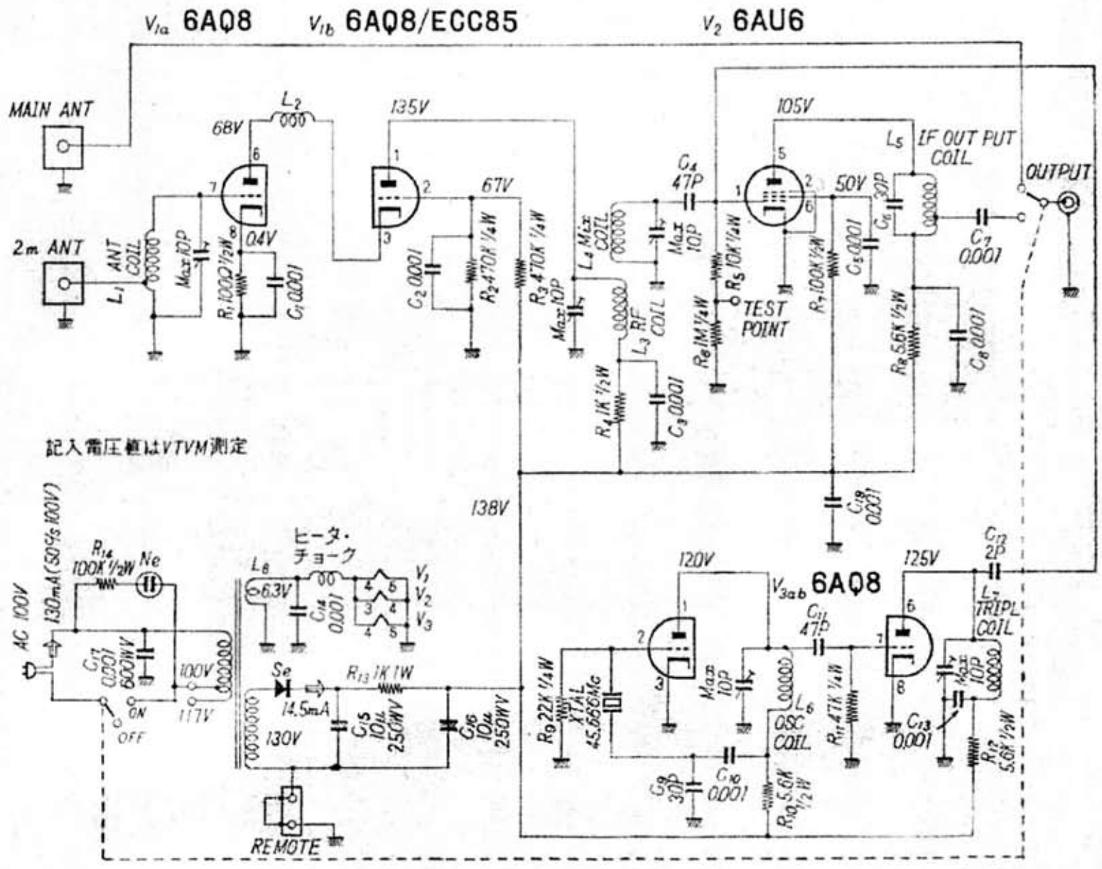
CC-2 形 クリコン の 全 回 路 図
