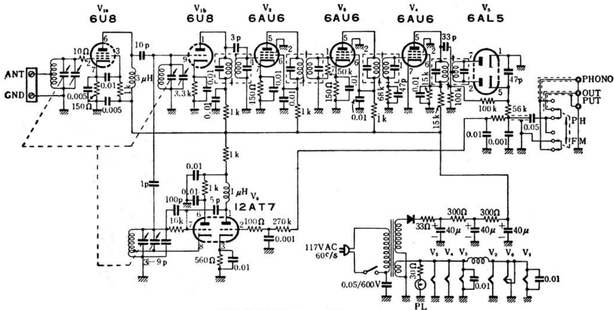
春日無線 FM-100 型チューナー
