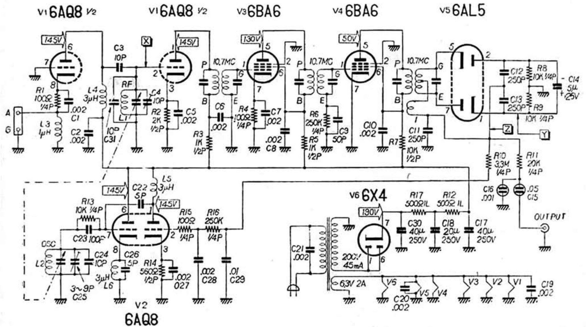
FM-110 形 FM チューナー配線図
