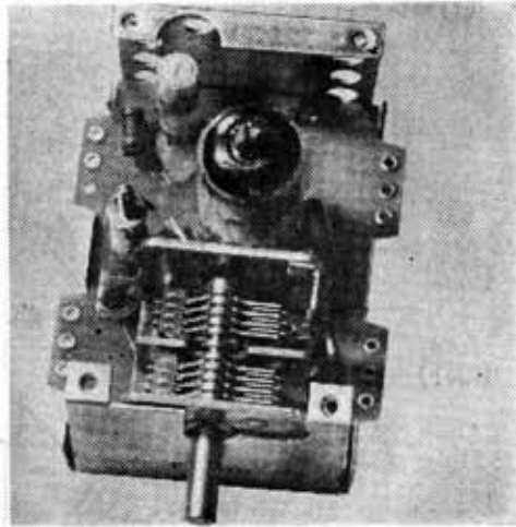
バリコン同調 FM フロントパック, トリオ FP-JD1
