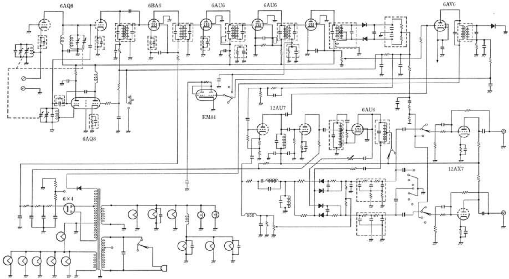
マトリックス方式FMステレオ・チューナー (トリオFX-2 1963年)
