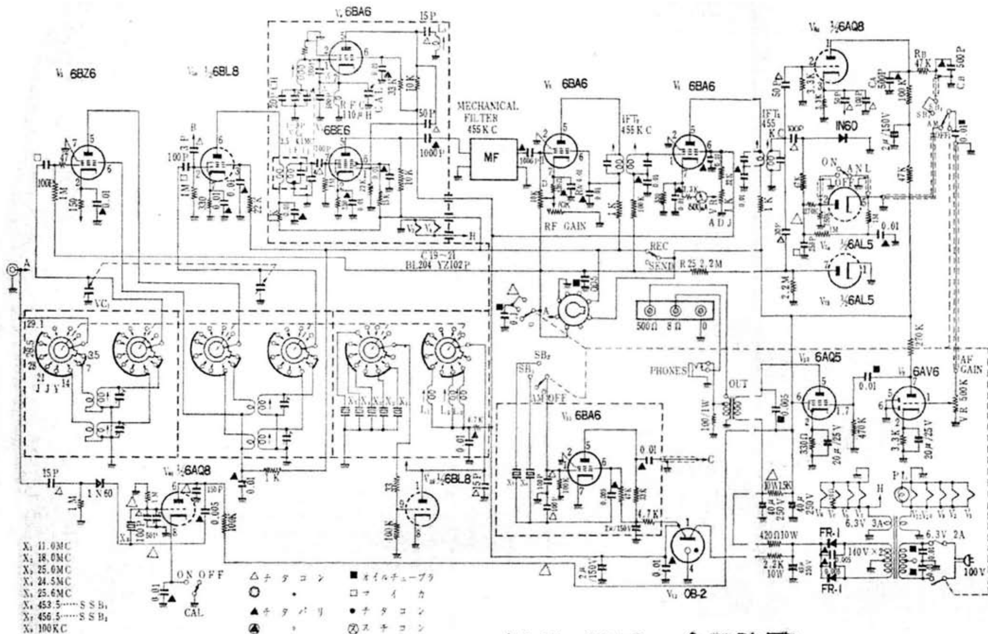
〈JR-600S 全回路図〉
