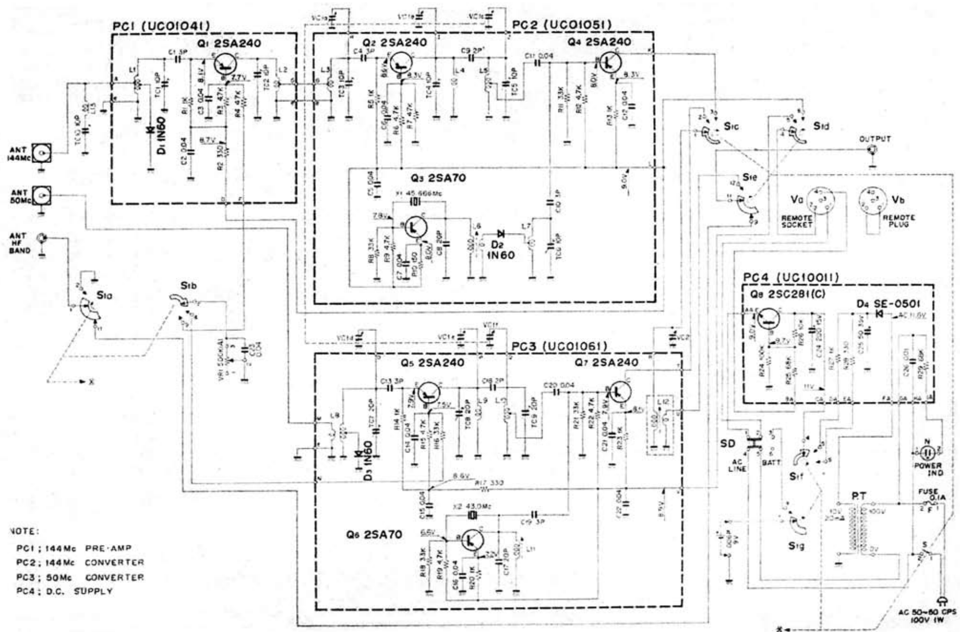
50/144Mc クリスタル・コンバータ「トリオCC-26」全回路図
