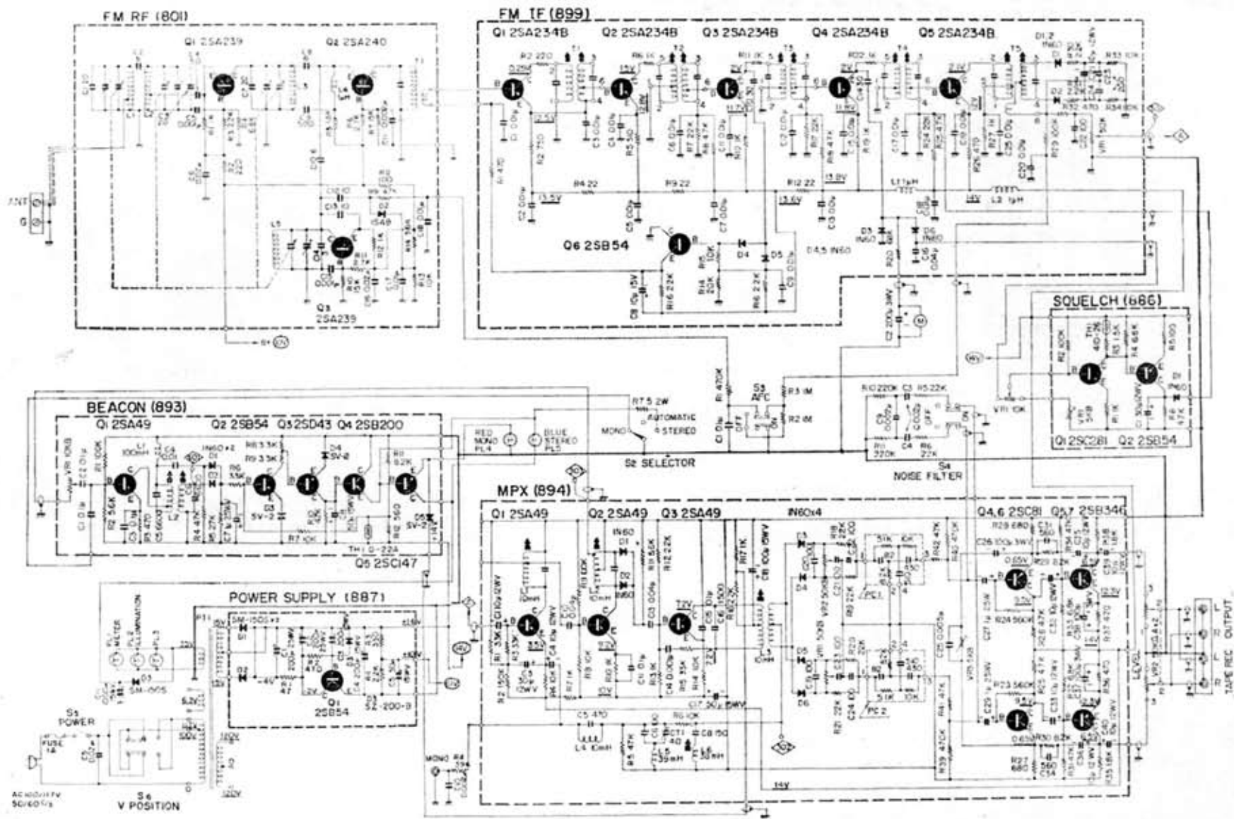
Trio FX-7T 形 FM チューナ全回路
