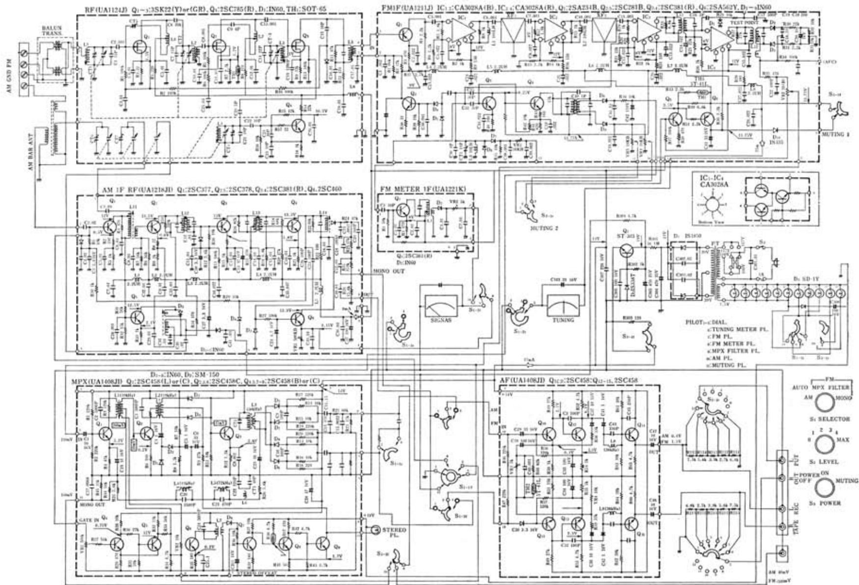
高級FMステレオ・チューナー（トリオKT-7000 1968年）
