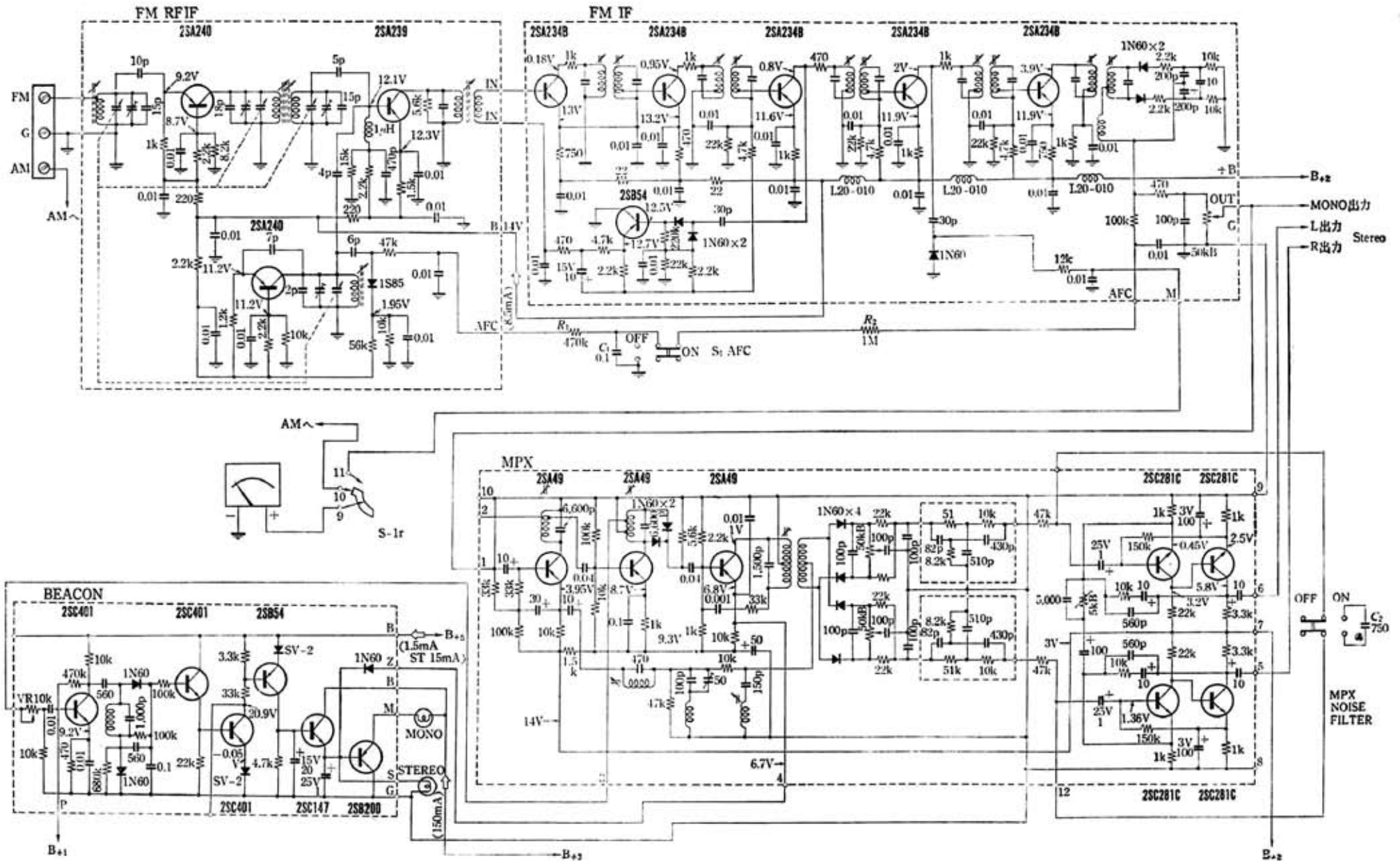
トリオ TW-410 型 FM チューナー部およびステレオ復調部回路図
