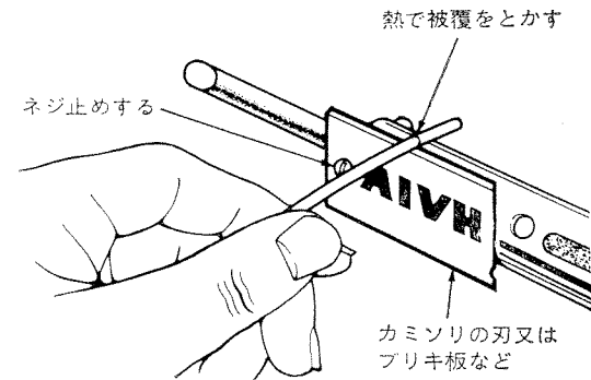
第9図 リード線のむき方
