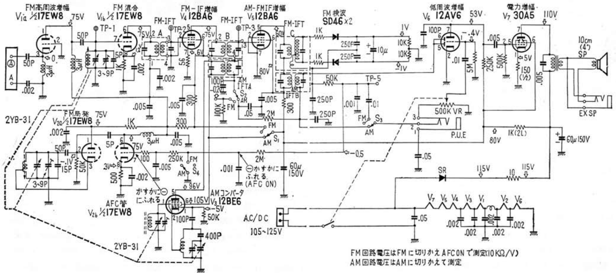
ユニオン FA-700形 FM/AM ラジオの回路
