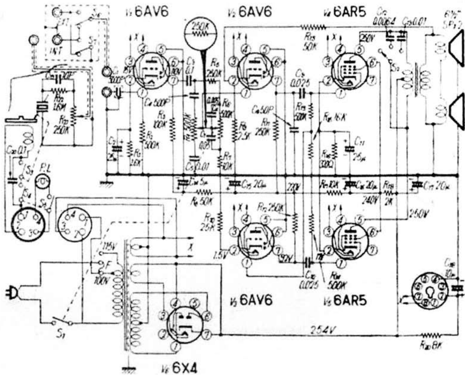
3 スピード卓上電蓄 E-13 型
