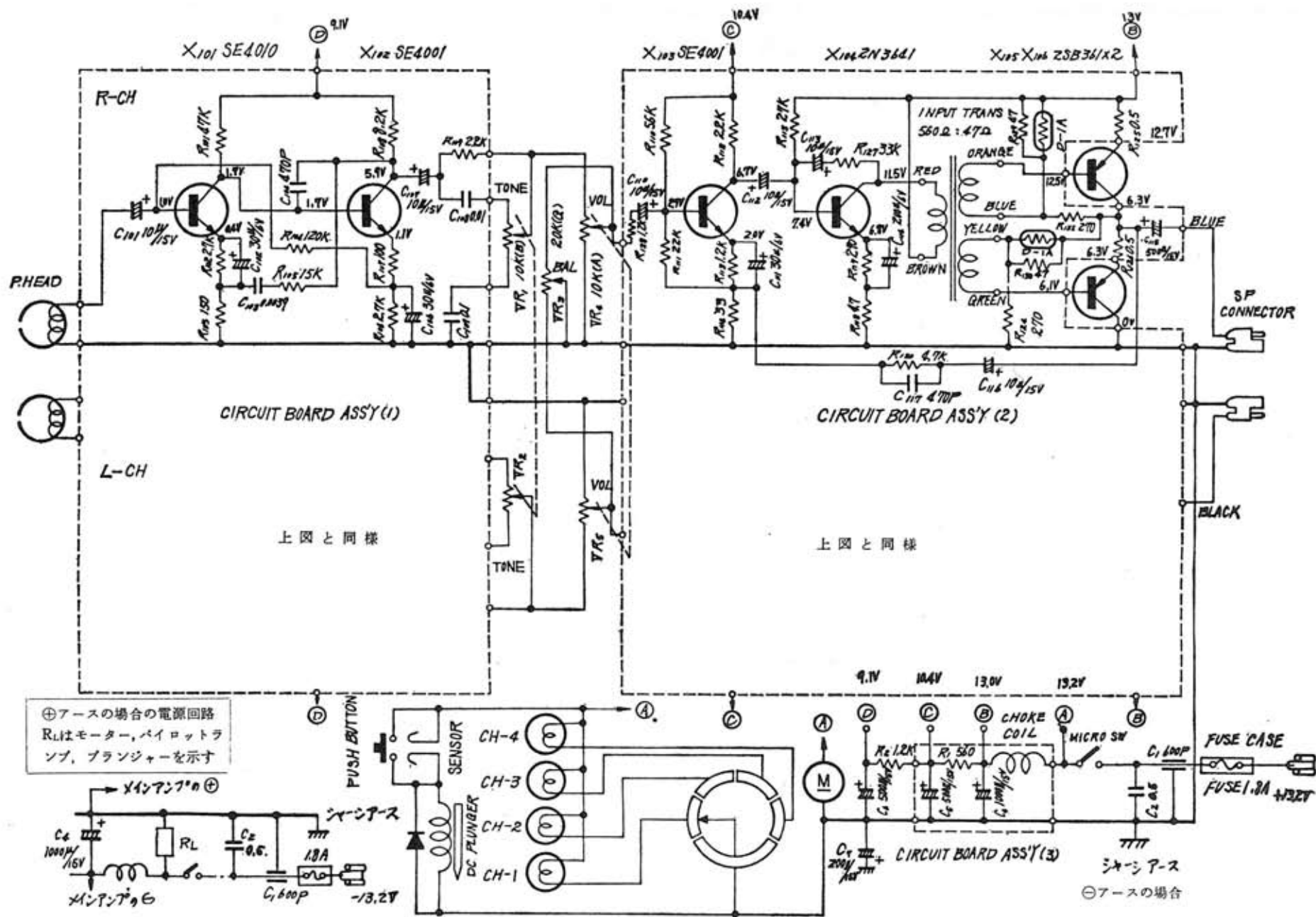
「ビクター」CAR-300 回路図
