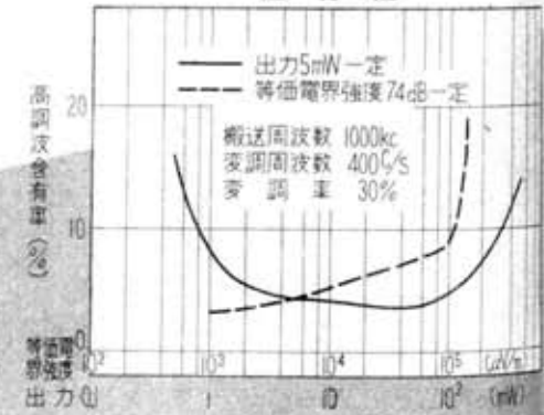
歪特性
