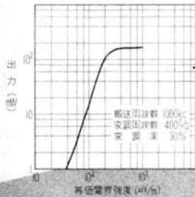
出力特性
