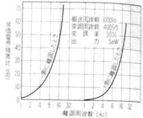
自動利得調節特性
