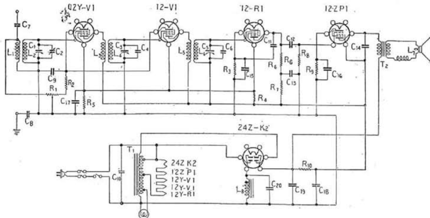
5A-10型 配線圖並に部分品定數
