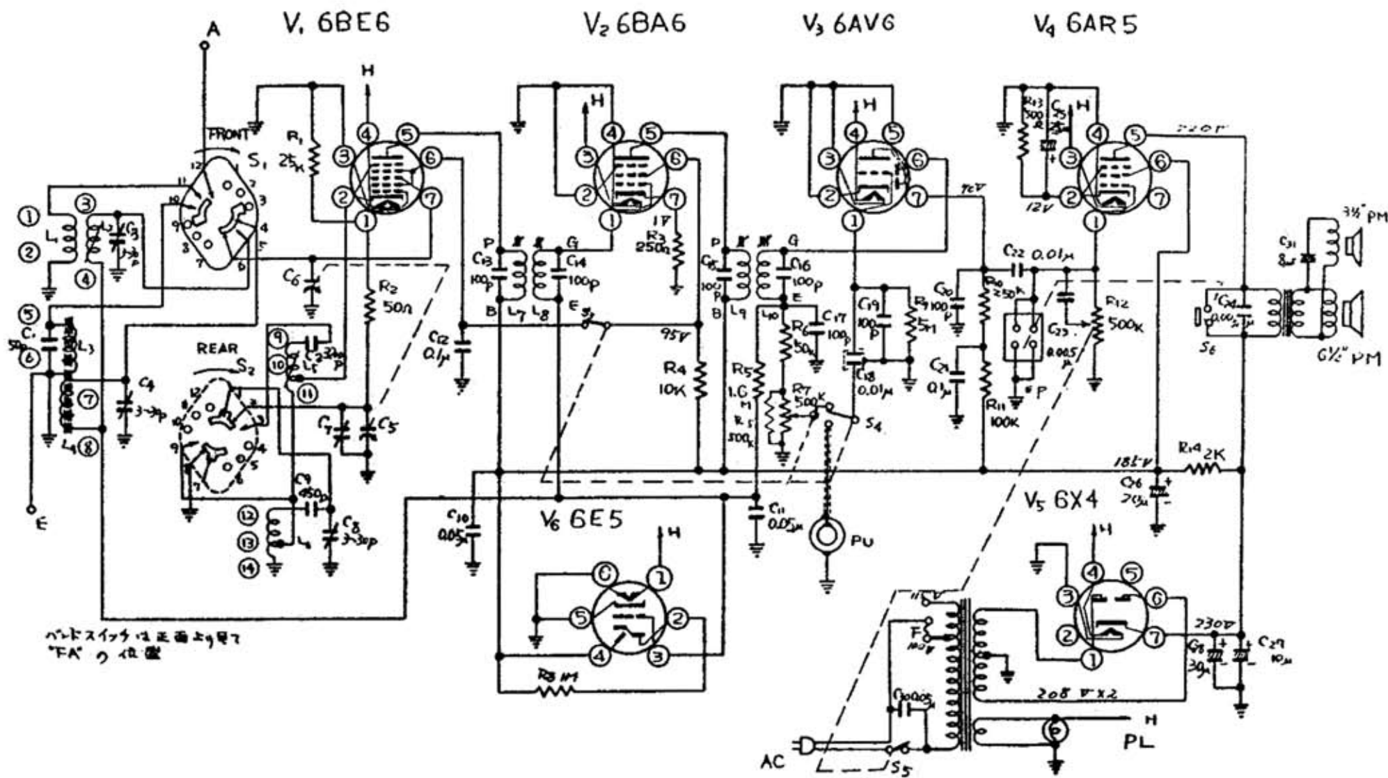
6A-2209型 配線図
