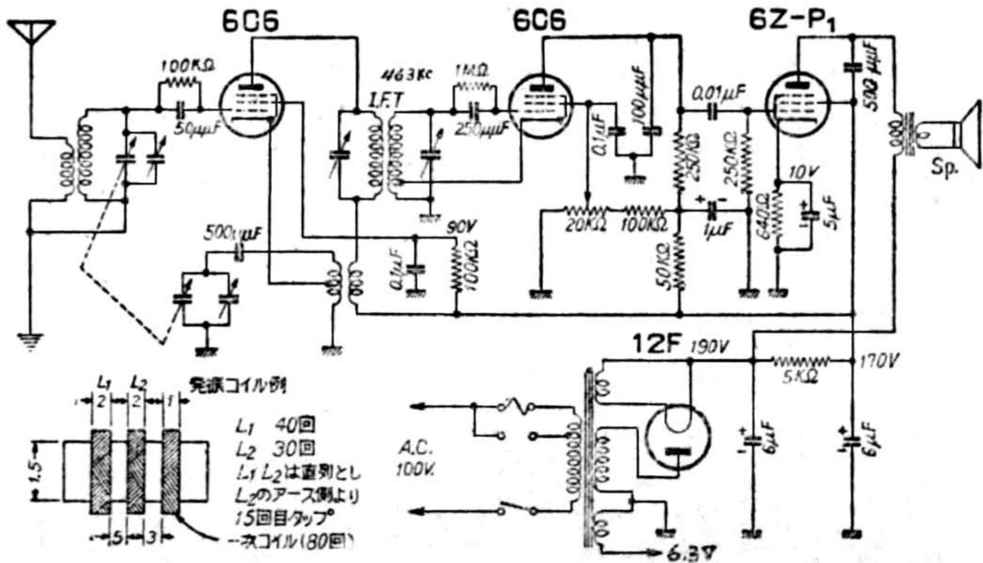
日本ビクター製 4R-1型 4球式スーパーヘテロダイン受信機
