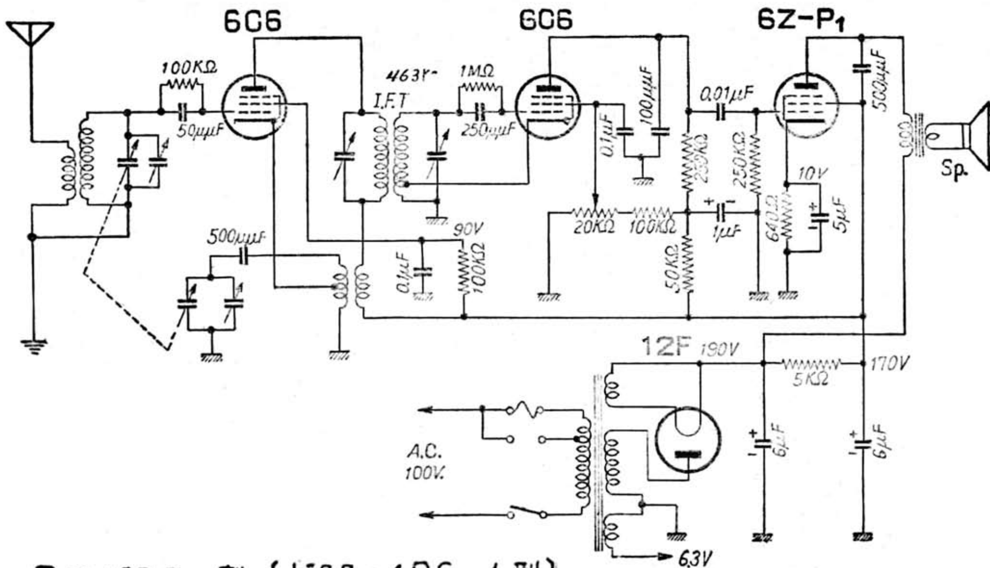
日本ビクター製〔ビクター-4RS-1型〕
