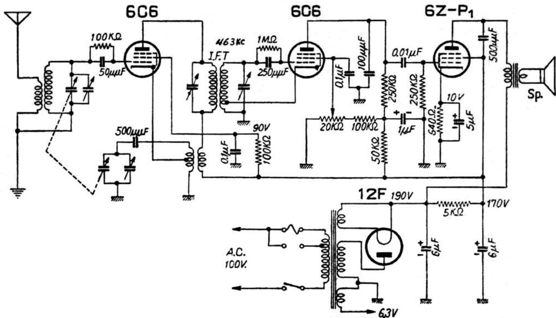
日本ビクター製 [ビクター4RS-1型] 4球式スーパーヘテロダイン受信機
