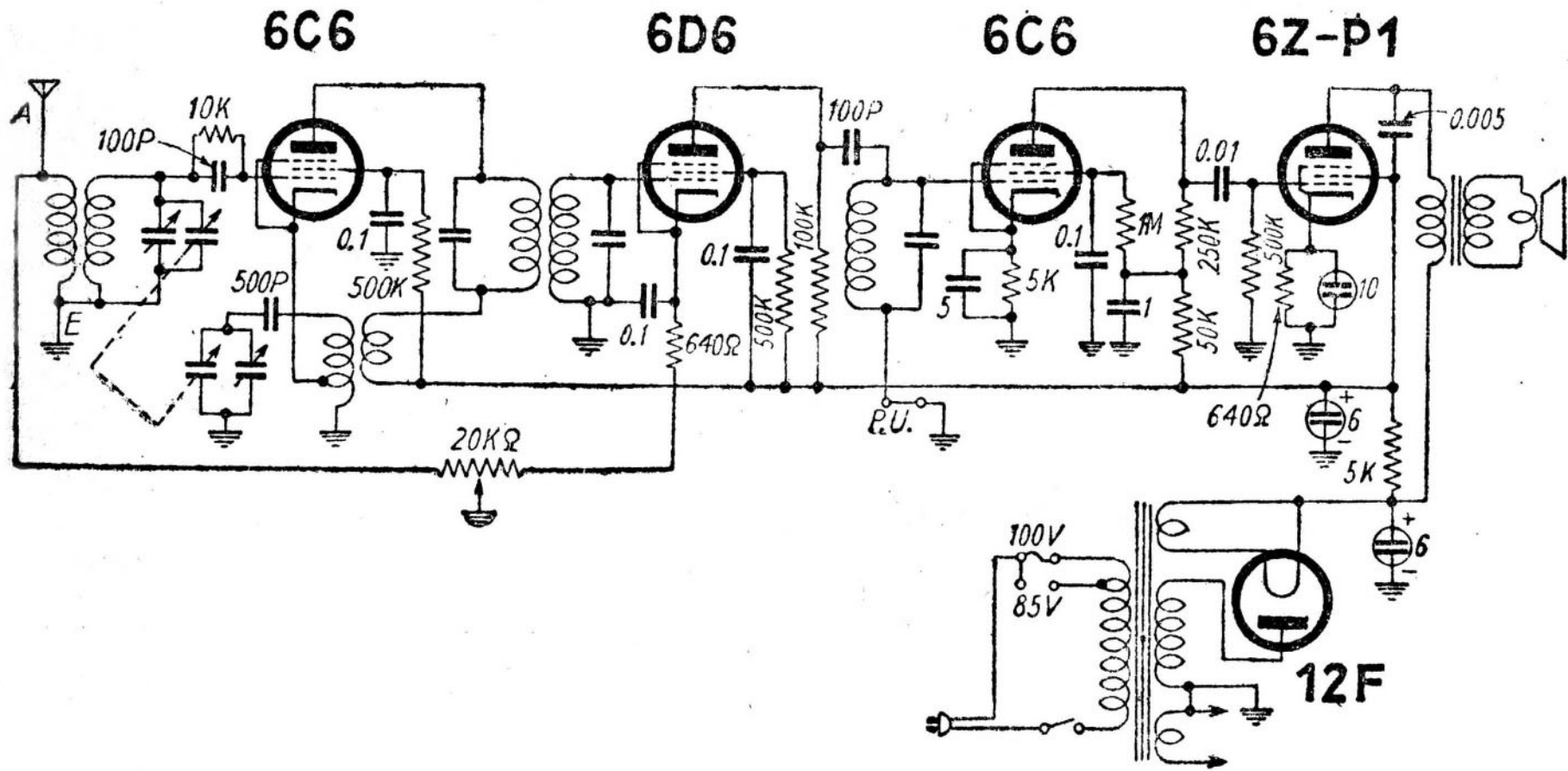
日本ビクター-5RS-2型5球スーパー
