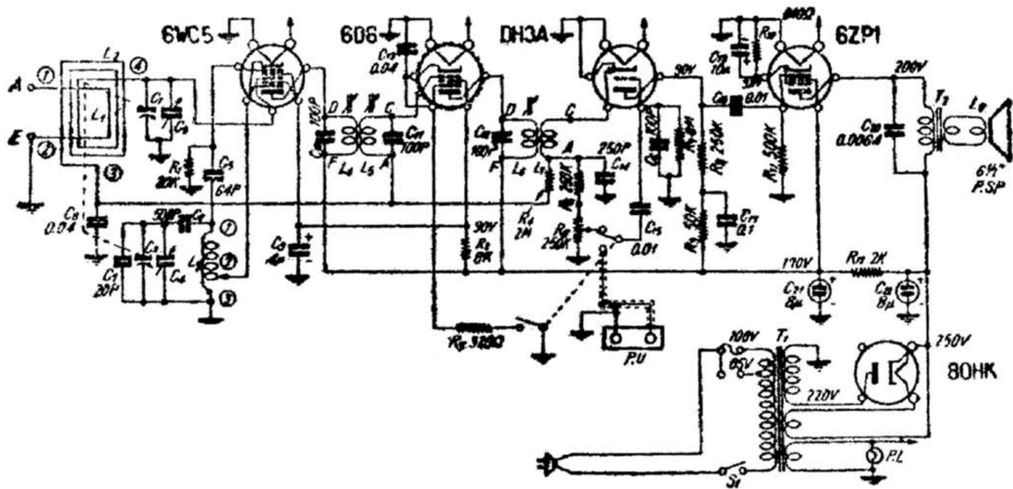
5RS-4型
