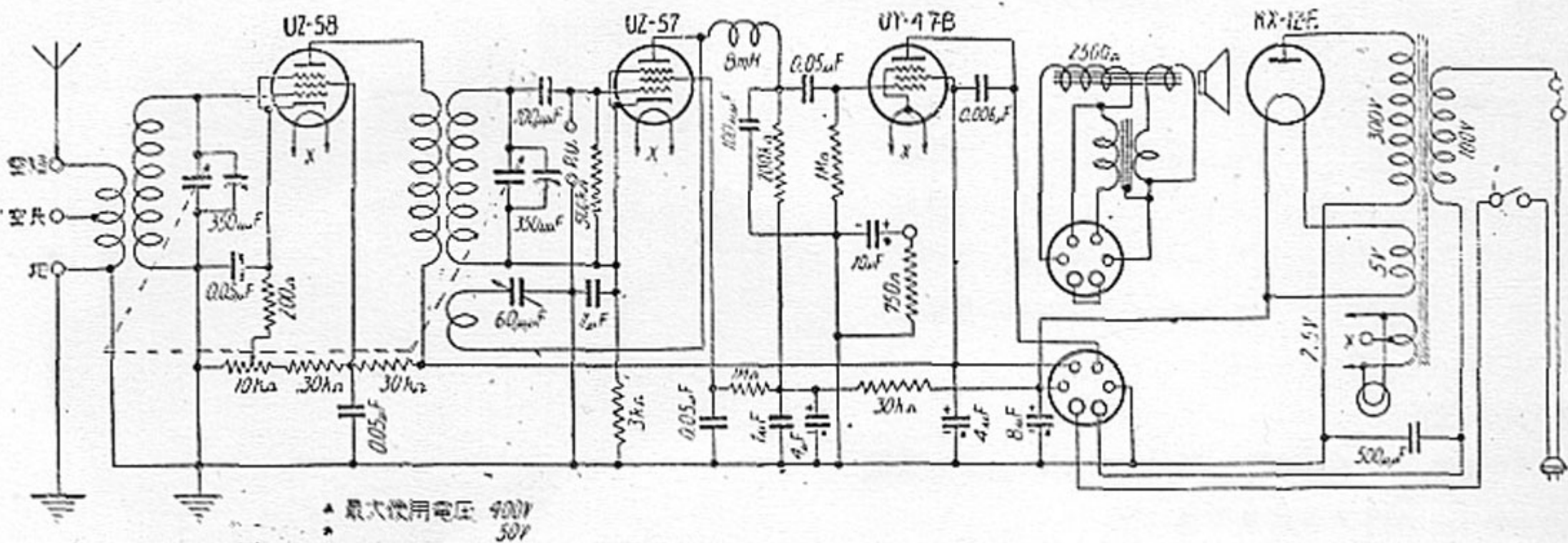
第 1 圖 [解剖した "E-11 號型" 受信機の回路結線圖.]
