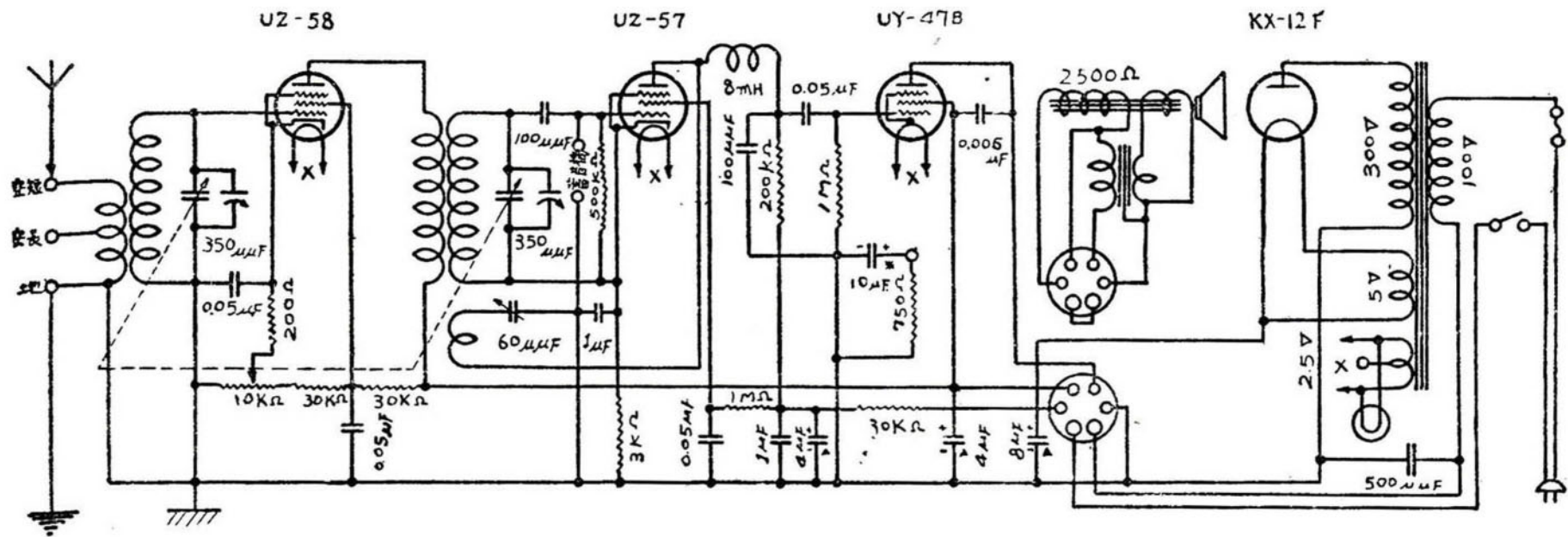
テレビアン E-11 號受信機回路接続圖
