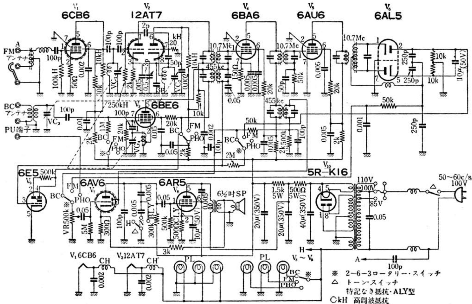
山中電機 FS-10 型 AM-FM 受信機
