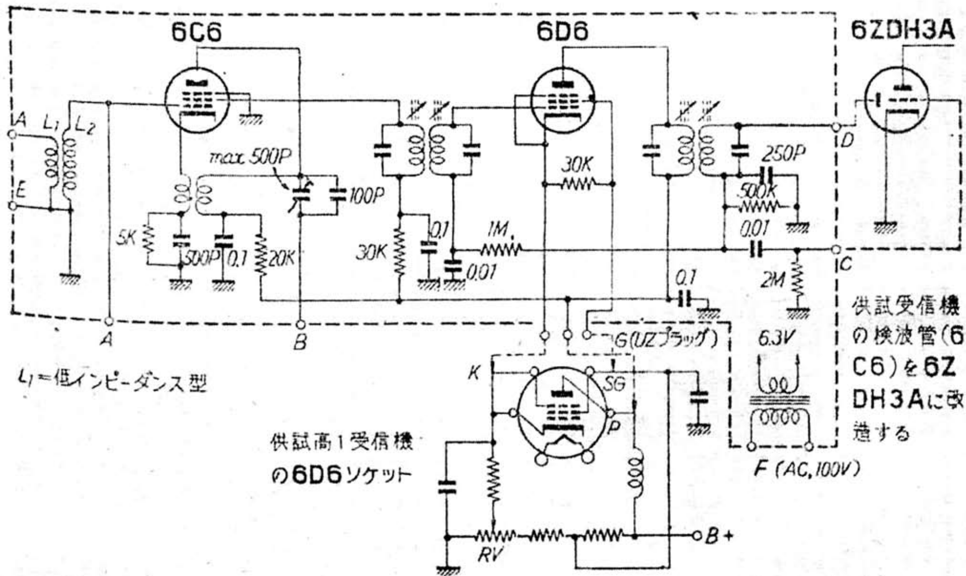
テレビアン・スーパー・ヘッド H-1型回路図
