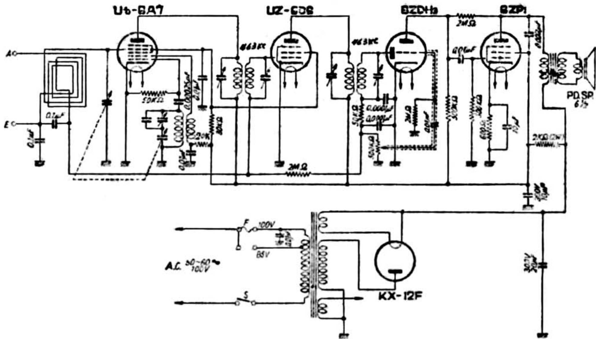
山中電機製 テレビアン R-52 號 5 球式スーパーヘテロダイン受信機
