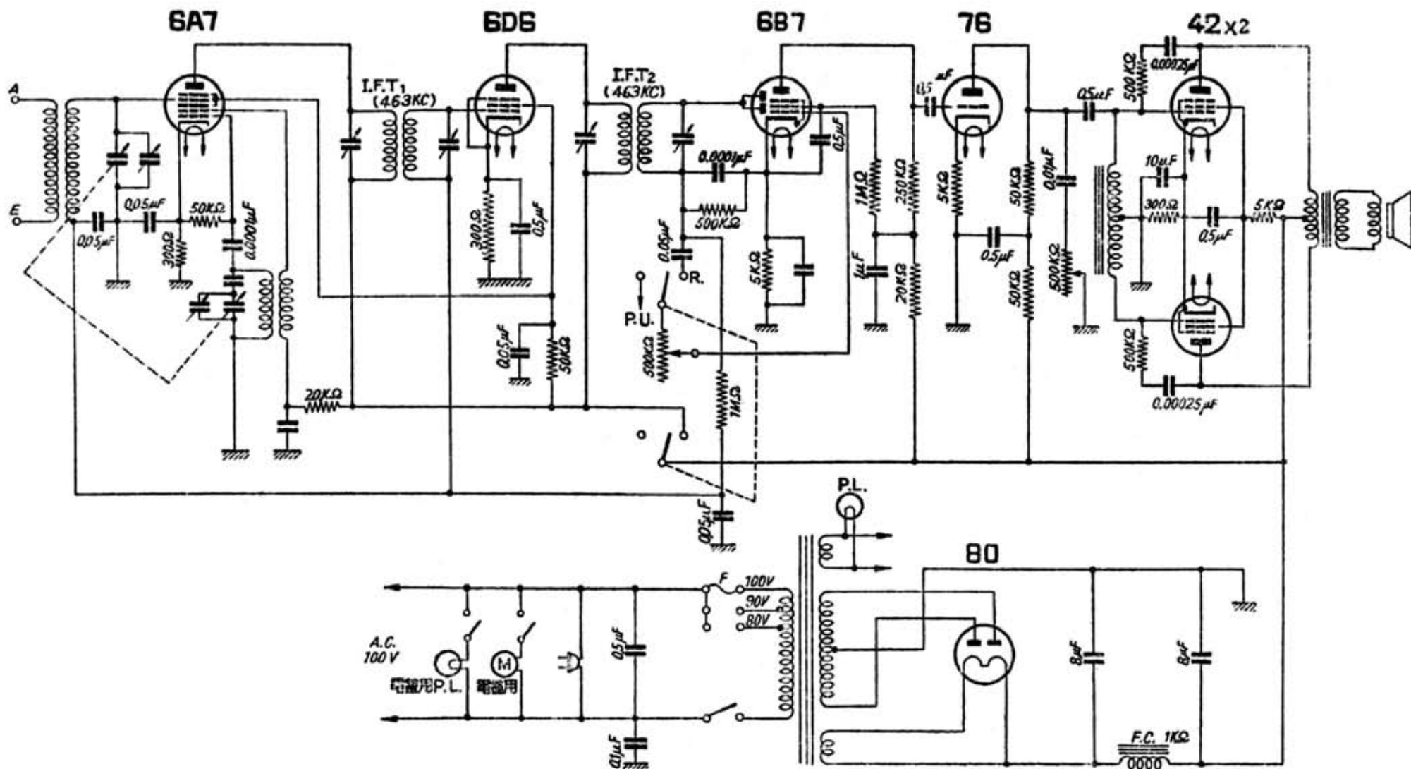
山中電機製 [テレビアン110型] 7球スーパーヘテロダイン受信機
