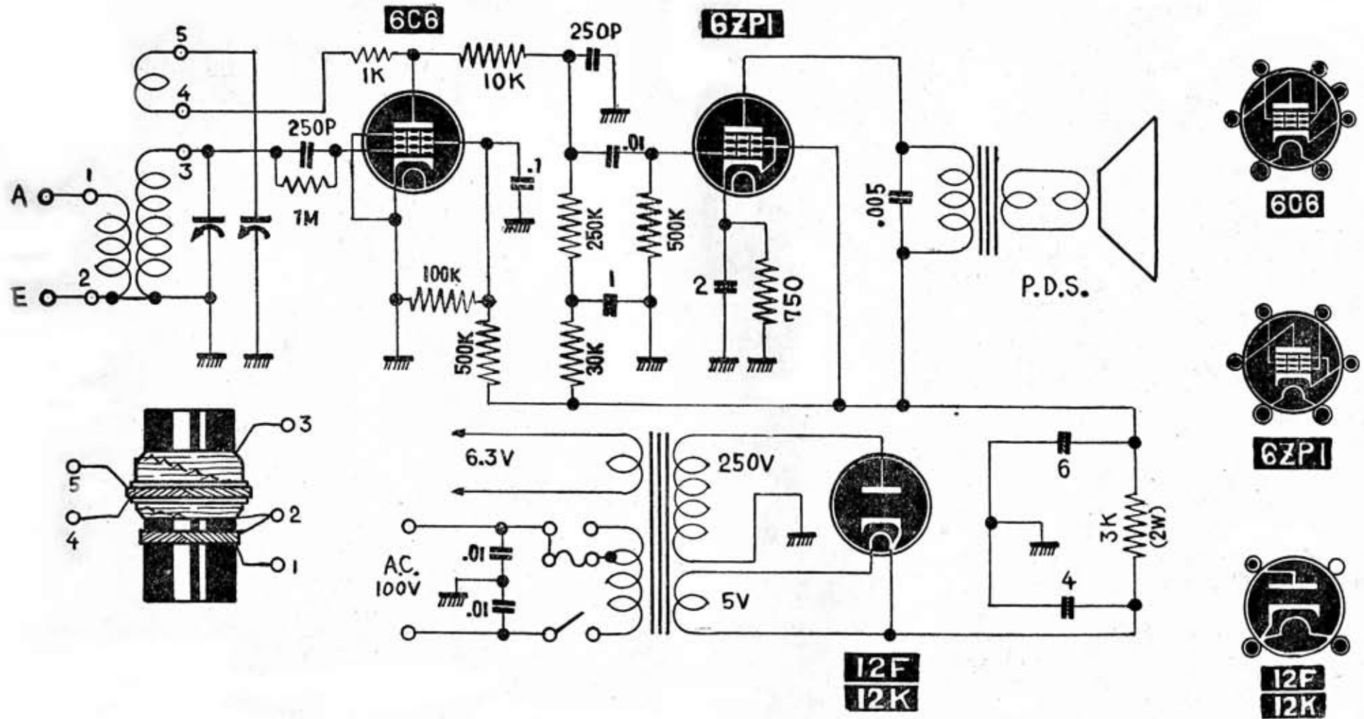
回路圖 No. 64 (3球式再生檢波) BR
